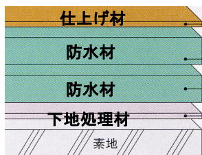
防水工程例
